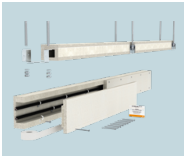
Brandschutzkanäle PYROLINE® Sun PV zur Leitungsverlegung in Flucht- und Rettungswegen
