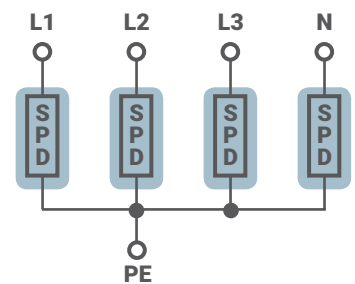
> Bild 6b: 4+0-Schaltung
