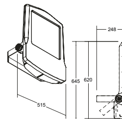
Mega Artikel-Nr. 60809... / 60810...
