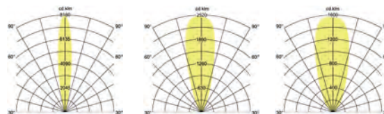
Art.-Nr. 14037223
