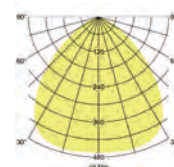
Mega Artikel-Nr. 60809... / 60810...
