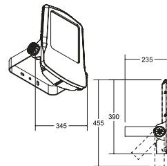
Mini Artikel-Nr. 60803... / 60804...
