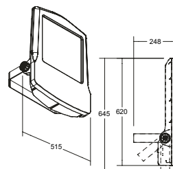
Maxi Artikel-Nr. 60807... / 60808...
