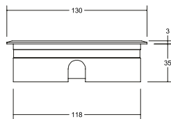
Art.-Nr. 14035223
