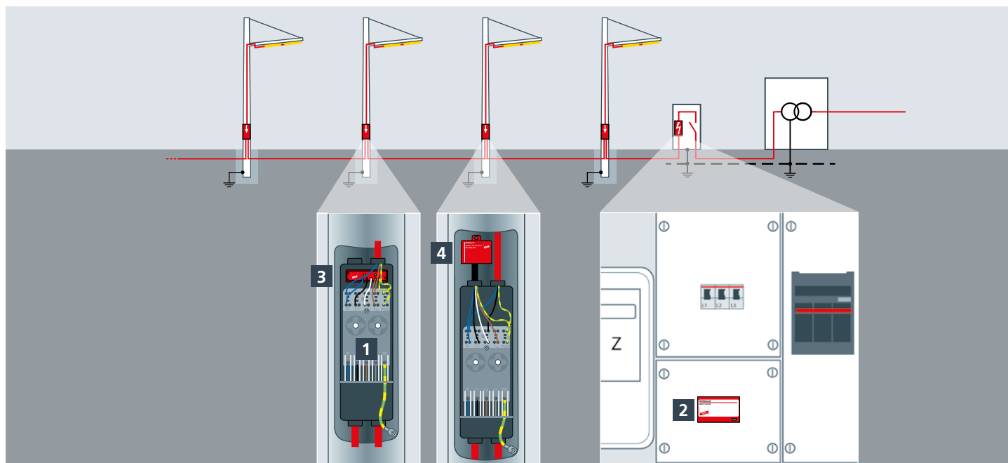
Die Überspannungs-Ableiter werden im Mast Sicherungskasten und in den Kabelverteilern der Einspeisung eingebaut.
