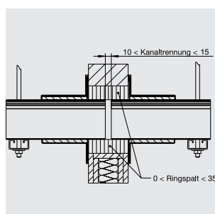
Kanal getrennt Wandöffnung \geq Kanalquerschnitt
