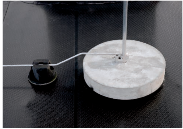
Bild 2: Fangstange mit Standfuß
