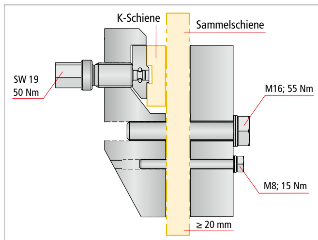
Klemmfestpunkt montiert auf Sammelschiene und eingebrachter KurzschlieÙschiene
