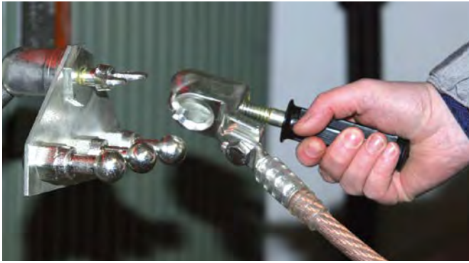
Erdanschlussplatte mit Kugelfestpunkten und Kugelkopfhabe mit Handgriff aus Kunststoff.
